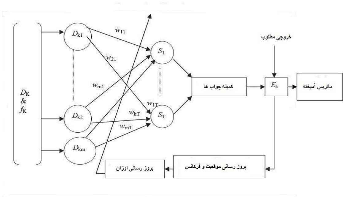
شکل ۴. الگوریتم بت
