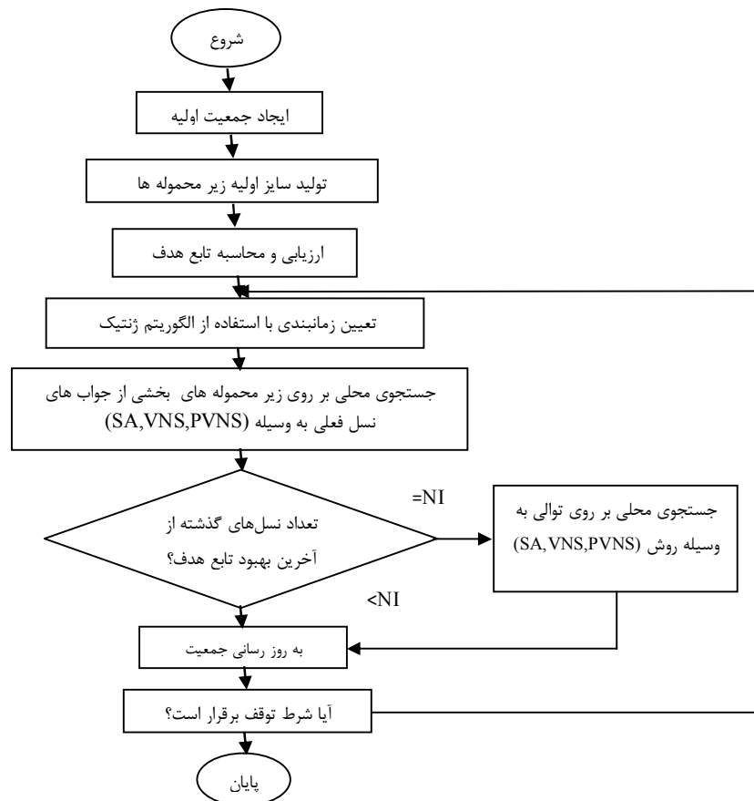
شکل ۲. شمایی از رویه بهینه‌سازی الگوریتم‌های پیشنهادی
