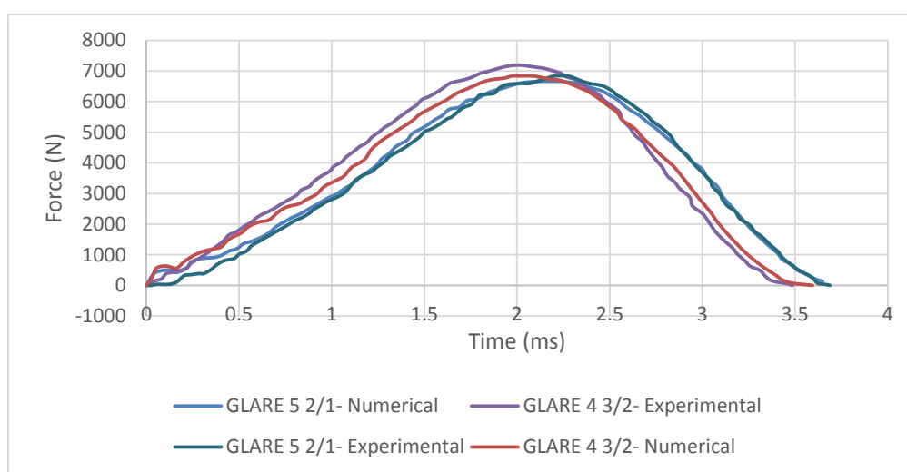
شکل ۸. مقایسه نتایج عددی و تجربی تاریخچه نیرو - زمان برای گلر ۱/۲ و ۲/۳ تحت ضربه با انرژی ۱۸ ژول
