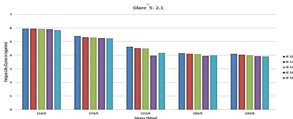
شکل ۹. نتایج خستگی پس از ضربه برای گلر ۱/۲
