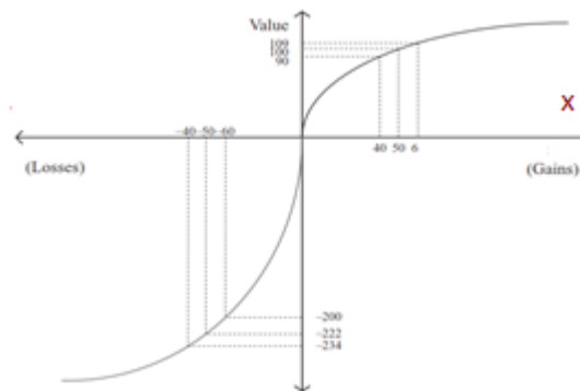
شکل ۲. یک تابع ارزش (سیگموئید) با در نظر گرفتن این سه اصل ارزش نظریه چشم‌انداز کاهنمن و تیورسکی ۱ (۱۹۹۲، ۱۹۷۹)
