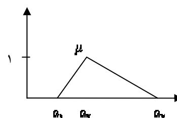
شکل ۱. عدد فازی \tilde{A} = (a_1, a_r, a_r)
