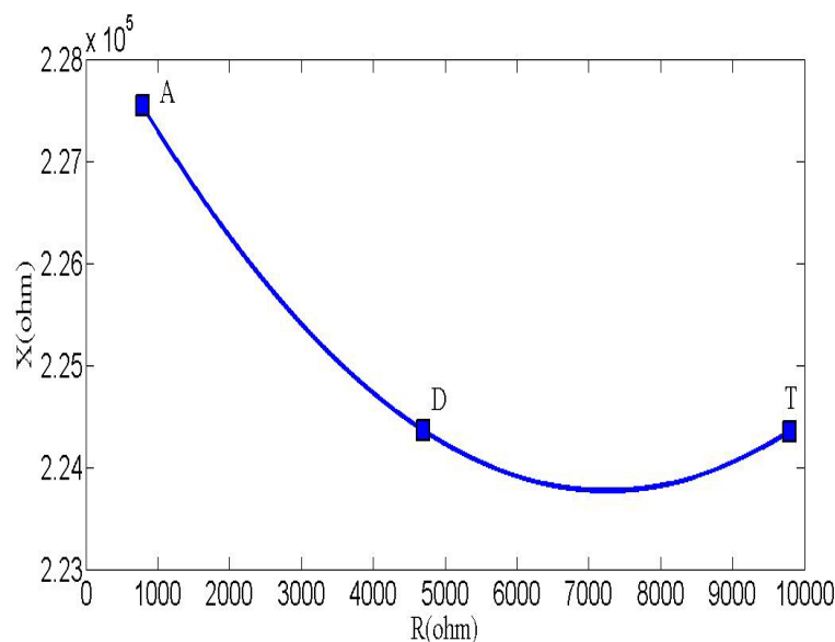
شکل ۱۸. منحنی تغییرات راکتانس پروب برحسب مقاومت پروب در بازرسی لوله فولاد زنگ‌زن برای موقعیت‌های مختلف
