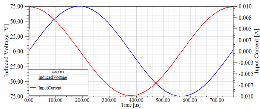
شکل ۹. منحنی ولتاژ و جریان پروب در هوا (حالت اول)
