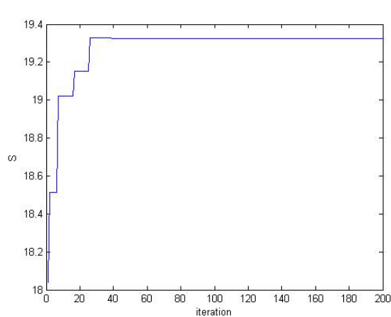
شکل ۷. نمودار تغییرات S بر حسب تکرار (لوله فولاد زنگ‌نزن)
