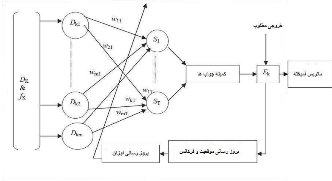
شکل ۴. الگوریتم بت
