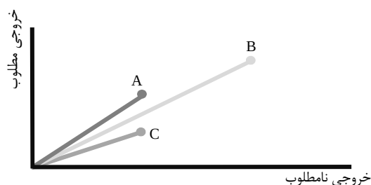
شکل ۱۰. میزان تاثیر اصل دسترسی پذیر ضعیف بر فضای امکان تولید سه واحد A, B, C
