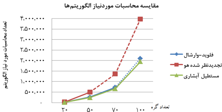
شکل ۳. عملکرد محاسباتی الگوریتم‌های مستطیل آبشاری، فلوید-وارشال و ماتریس تجدیدنظر شده هو برای شبکه‌های مختلف
