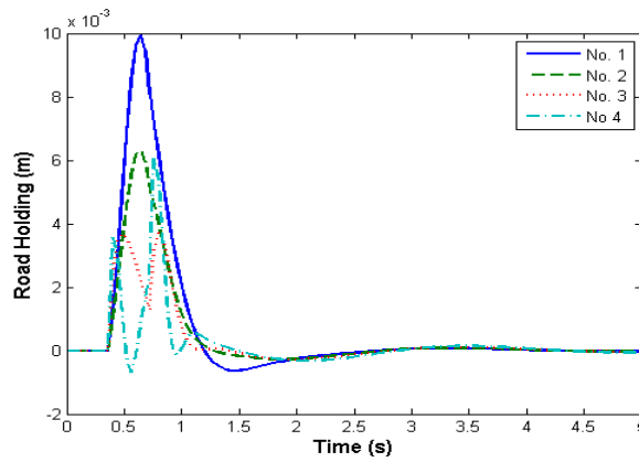
شکل ۱۹. نمودار اختلاف ورودی جاده و تایر بر حسب زمان؛ بهینه شده توسط روش الگوریتم ژنتیک در ۴ نقطه طراحی مختلف
